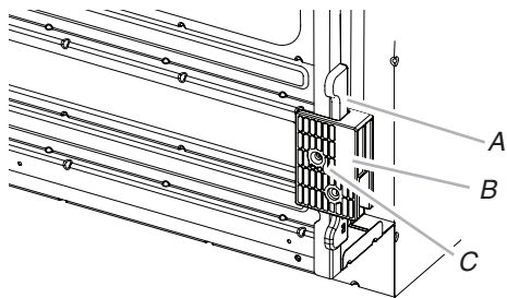
A. Cale d'espacement B. Pied C. Vis n° 8-18 x \frac{3}{8} " (9,5 mm)
