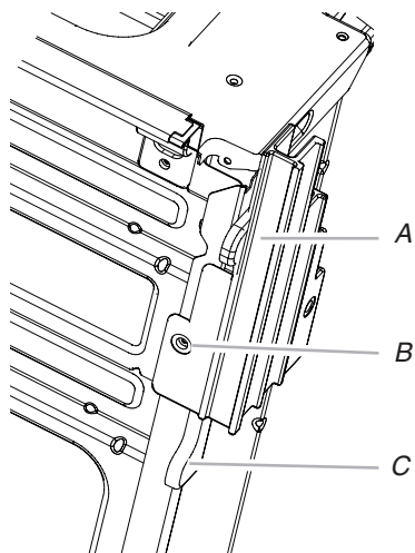
A. Pied avant B. Vis n° 8-18 x \frac{3}{8} " (9,5 mm) C. Cale d'espacement
