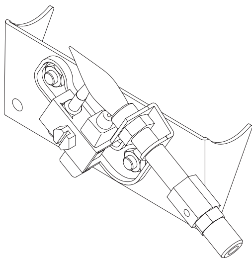
Fig. 20 - Patrón correcto de llama piloto
