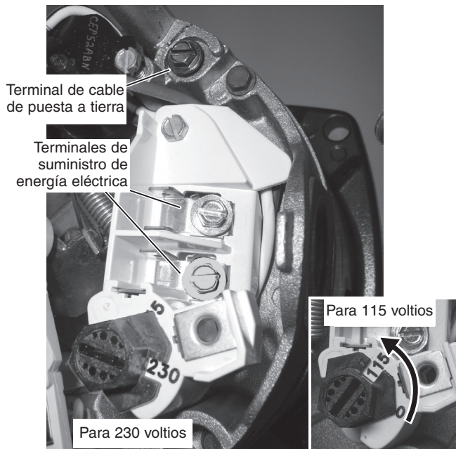
Figura 4: Configuración de tensión a 230 voltios, tipo cuadrante; gire el cuadrante hasta que marque 115 voltios. Introduzca una herramienta en la ranura para hacer girar el cuadrante.
