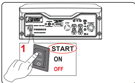
Fig 9 Arranque eléctrico
