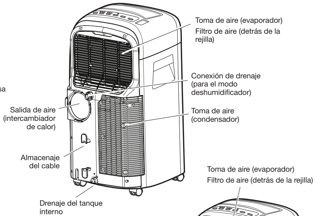
Vista posterior (modelos de una sola ventilación)
