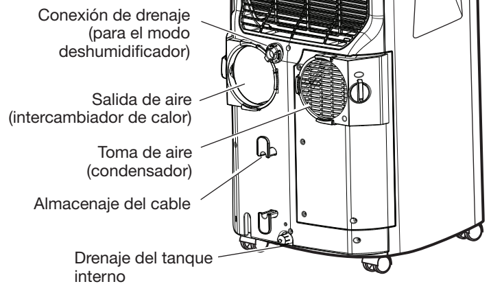
Vista posterior (modelos de ventilación doble)
