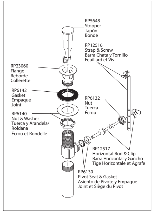
RP26533 Metal Pop-Up Assembly Less Lift Rod Ensamble de Metal del Desagüe Automático Menos Barra de Alzar Envió Mecánico en Metal Sans la Tige de Manoeuvre
