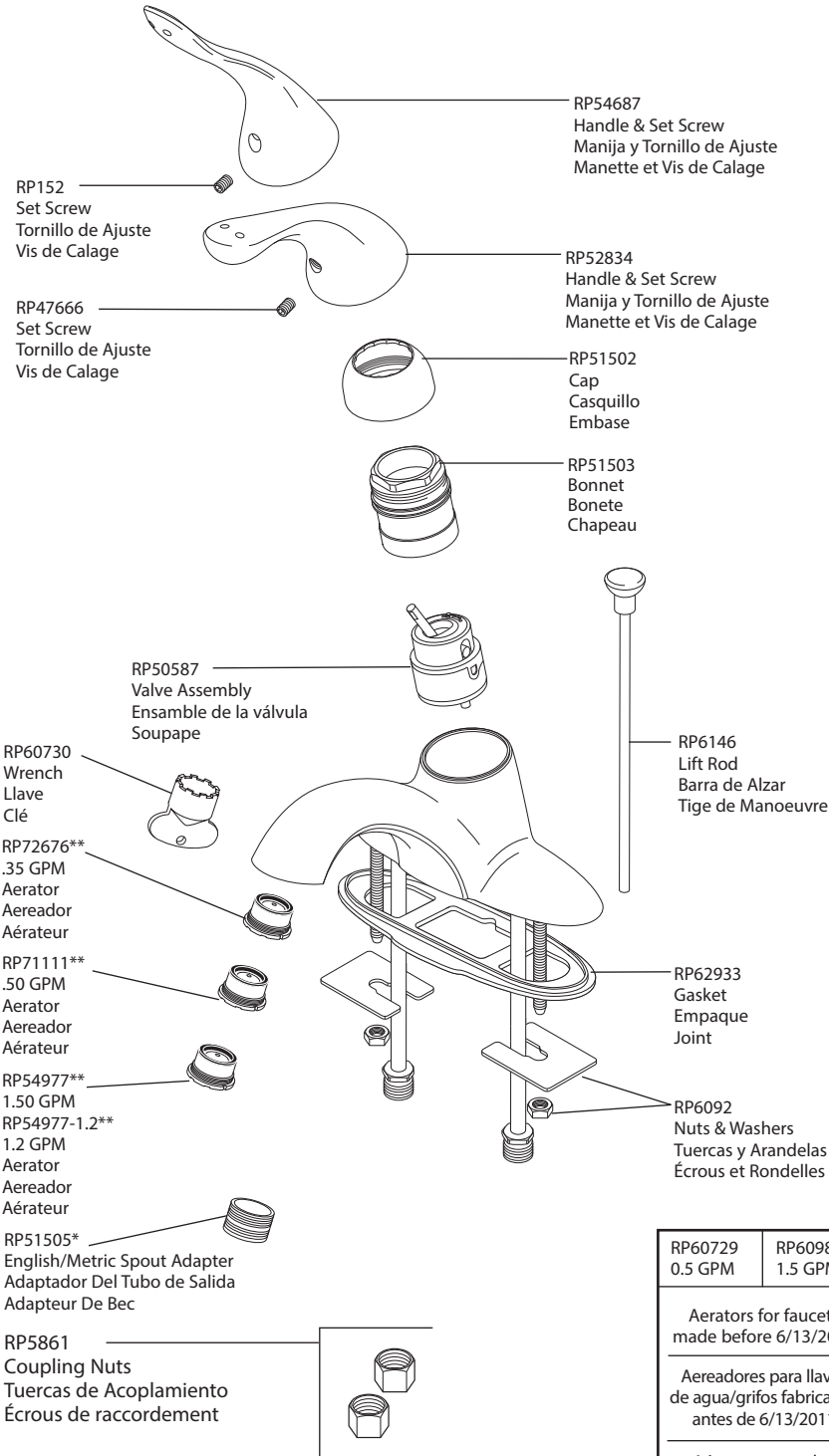
RP26533 Metal Pop-Up Assembly Less Lift Rod Ensamble de Metal del Desagüe Automático Menos Barra de Alzar Envió Mecánico en Metal Sans la Tige de Manoeuvre
