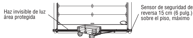
Enfrentando la puerta desde el lado interno del garaje
