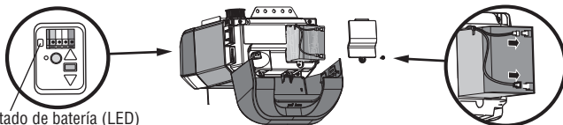
Estado de batería (LED)
