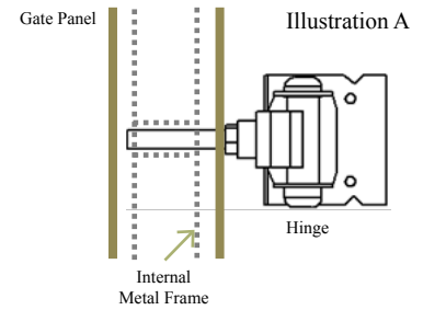
SimTek Hinge
