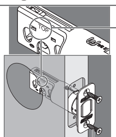
Figure A: Mortaise
