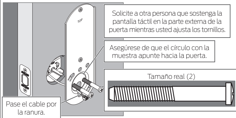
Figura B: Sin mortaja
