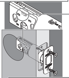
Figure A: Mortise
