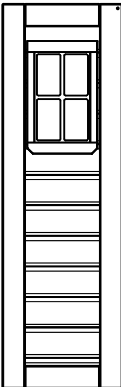
WP3 - PANEL IZQUIERDO LADO DERECHO DE LA (1) PARED - W2A01762 1 1/8"x12 5/8"x39 7/8" (27x320x1014)
