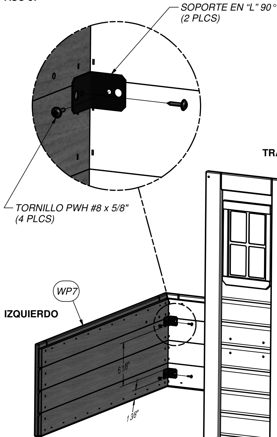
WP7 - PANEL DE PARED IZQUIERDA - W2A01766 (1) 1 1/8"x38 3/4"x13" (27x984x330)
