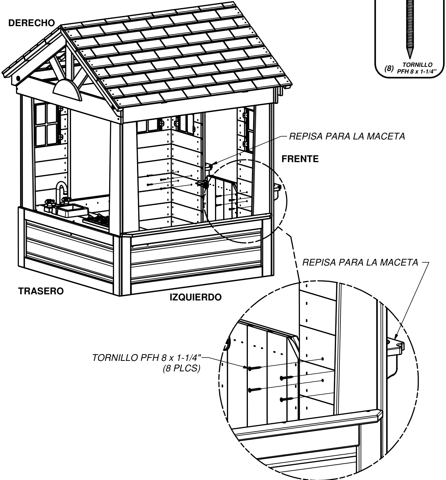
(2) - REPISA PARA LA MACETA - A6P00023
