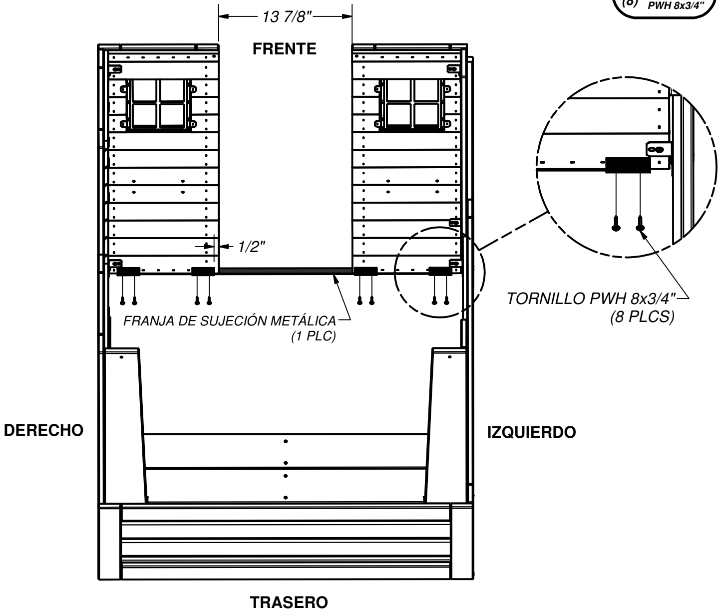
(8) TORNILLO PWH 8x3/4"
