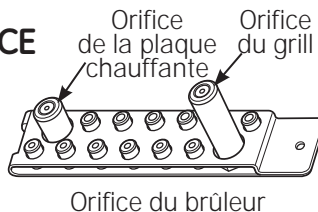
Orifice du brûleur
