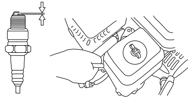
Figura 4-8. Bujía
