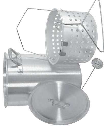
Modèle : 30BV Récipient de 28 l, crochet pour égoutter, panier, crochet de levage, couvercle et thermomètre
