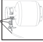
Queimador, manguera, regulador y válvula del tanque.
