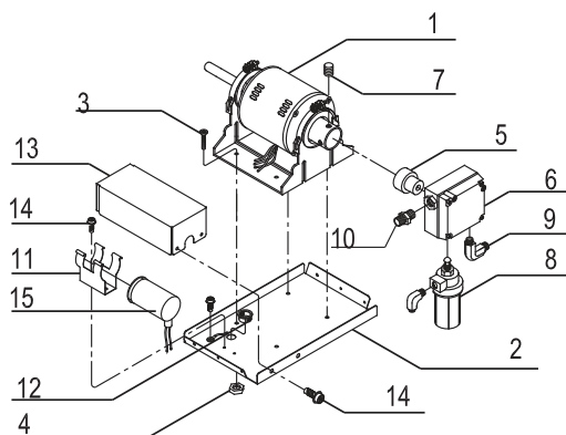
Figure 19. Moteur et pompe
