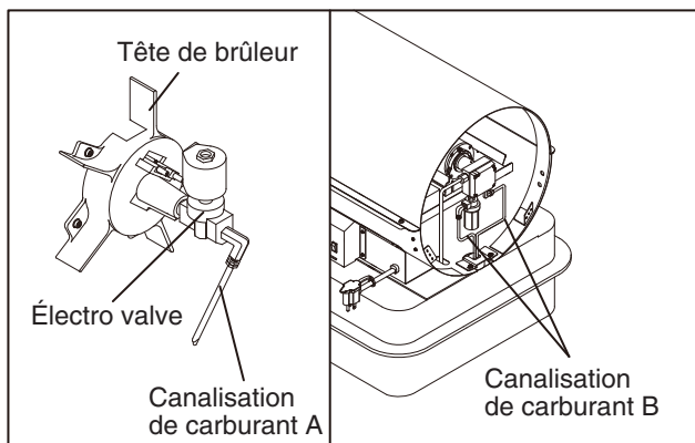
Figure 12. Serrer la canalisation de combustible
