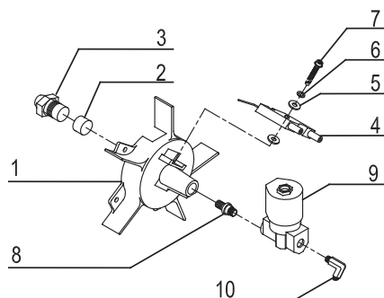
Figure 18. Tête de brûleur
