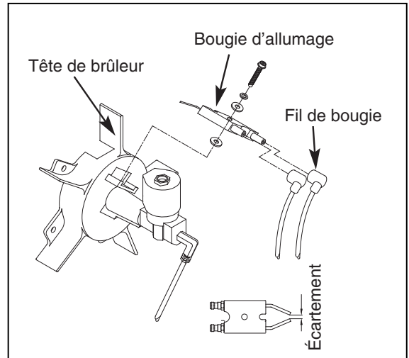
Figure 9. Bougie d'allumage
