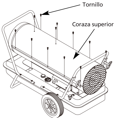
Figura 7. Desmontaje de la Coraza Superior
