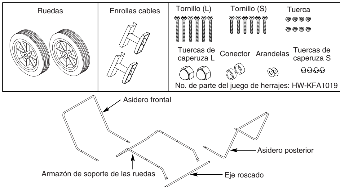
Figura 2. Identificación de los componentes
