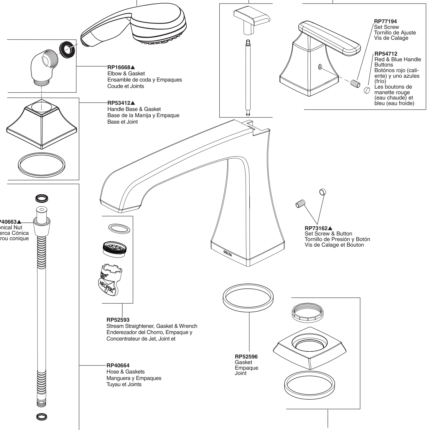
RP77196▲ Handle Base, Nut & Gasket Base de la Manija, Tuerca y Empaque Base, écrou et joint de manette
