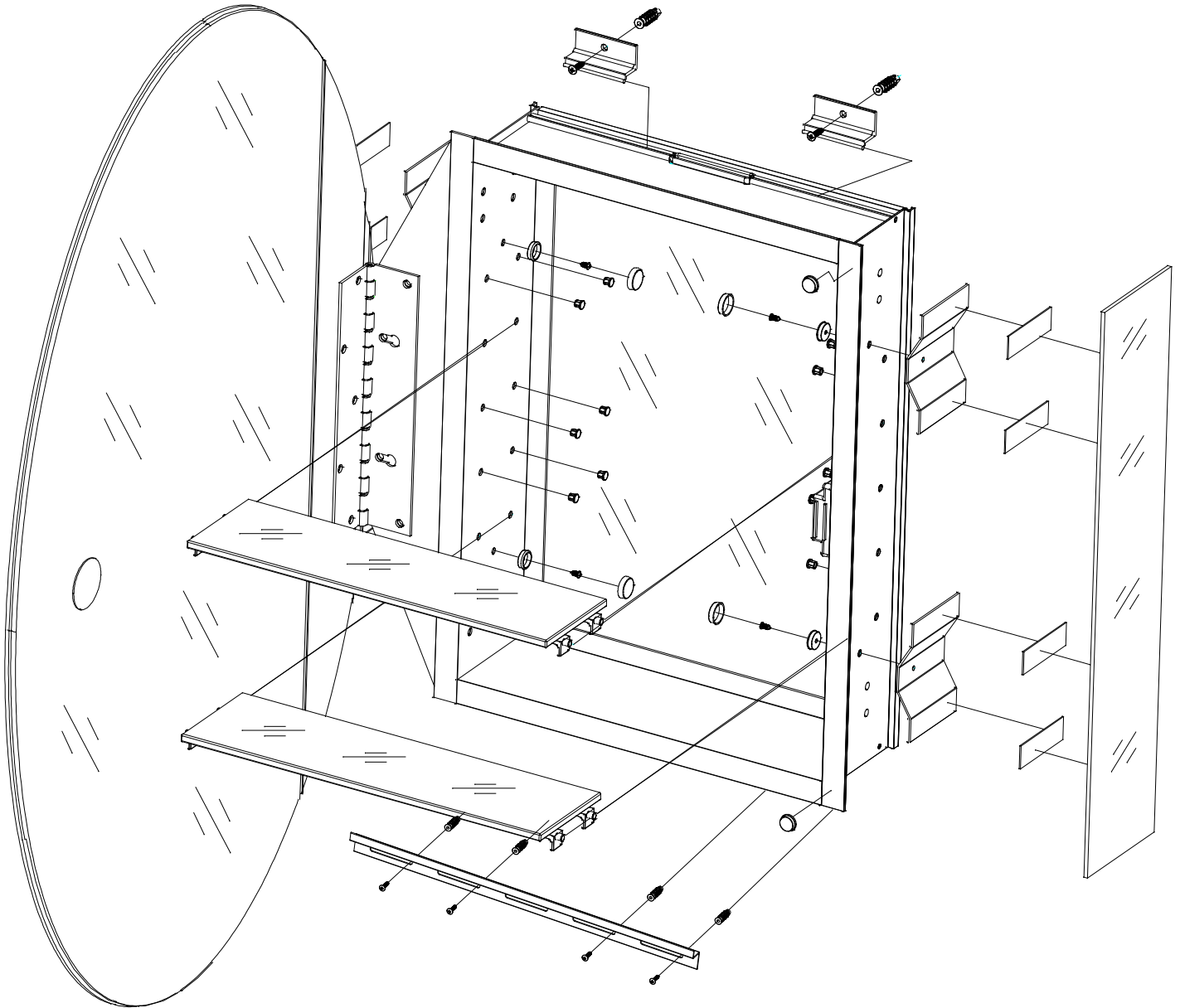
Explode view Vista explosiva
