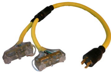
Twist lock adapter - 240V to six 120V outlets Adaptador de cierre por torsión de 240V a 6 salidas de 120V
