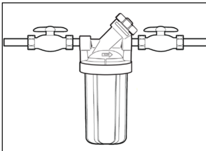
l'installation suggérée
