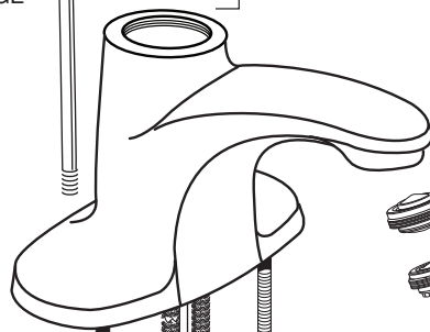
M964479-0070A AÉRATEUR (1,2 gpm)
