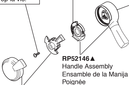
RP52147 ▲ Temperature Knob and Cover Perilla de la Temperatura y Cubierta Poignée de Réglage de Température
