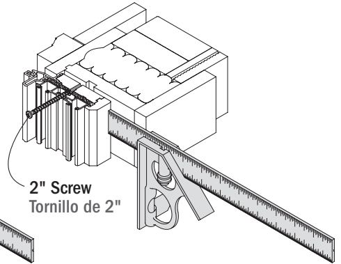
Tilt-Wash Double-Hung Window Ventana de doble guillotina inclinable para limpieza
