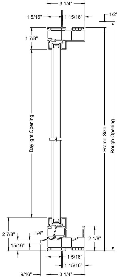
DP 35
