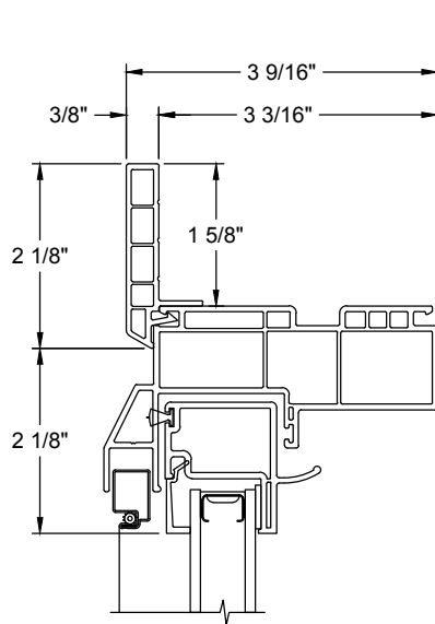
1 5/8" Flush Fin
