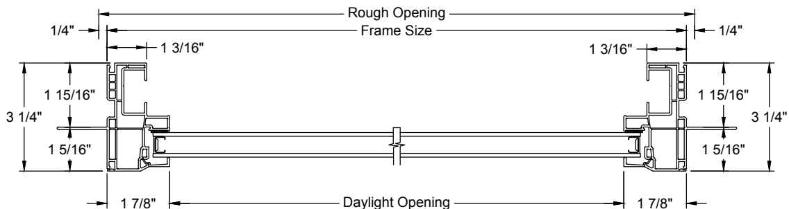
DP 35 / DP 50
