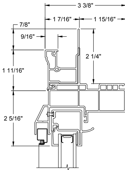
Brickmould
