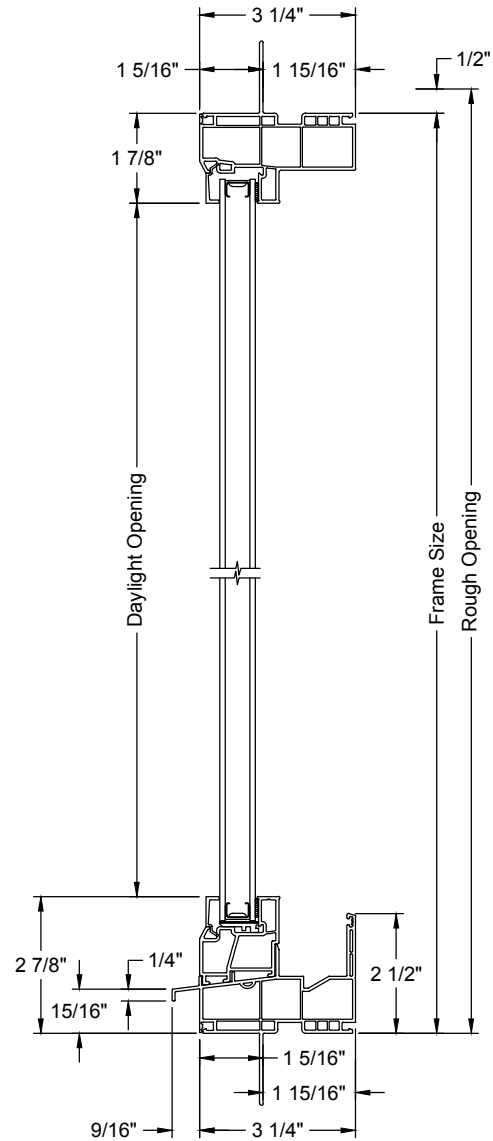
DP 50
