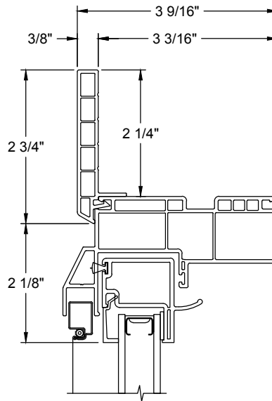
2 1/4" Flush Fin
