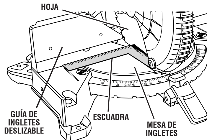
VISTA DE LA HOJA FUERA DE ESCUADRA CON LA GUÍA; SE REQUIEREN AJUSTES Fig. 17
