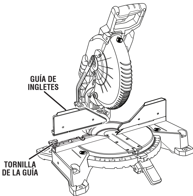
VISTA DE LA SIERRA DESDE ATRÁS CON LAS GUÍAS MIRANDO HACIA ADELANTE
