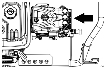
Figure 3-12. Déplacement de la pompe vers le moteur
