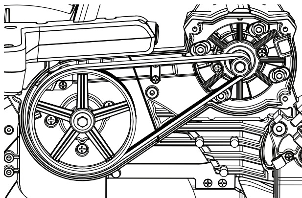
Figure 53. Courroie d'entraînement
