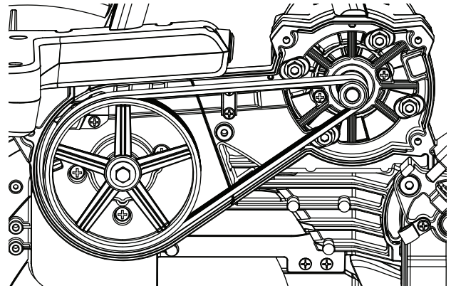
Figura 53. Polea motriz
