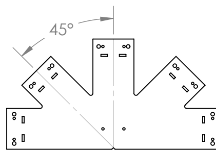
56644 12:12 Truss Base Fan
