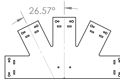
56643 6:12 Truss Base Fan
