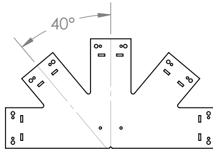
56620 10:12 Truss Base Fan
