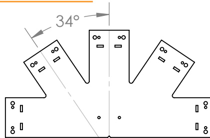
56619 8:12 Truss Base Fan
