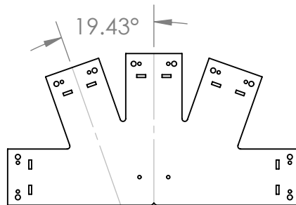
56642 4:12 Truss Base Fan
