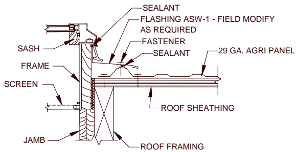
Detail A-A
