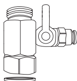
Valve en T d'alimentation en eau avec rondelle en caoutchouc (connexion 1/2")
