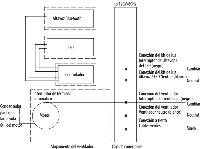
CABLEADO PARA 2 OPERACIONES DEL INTERRUPTOR
