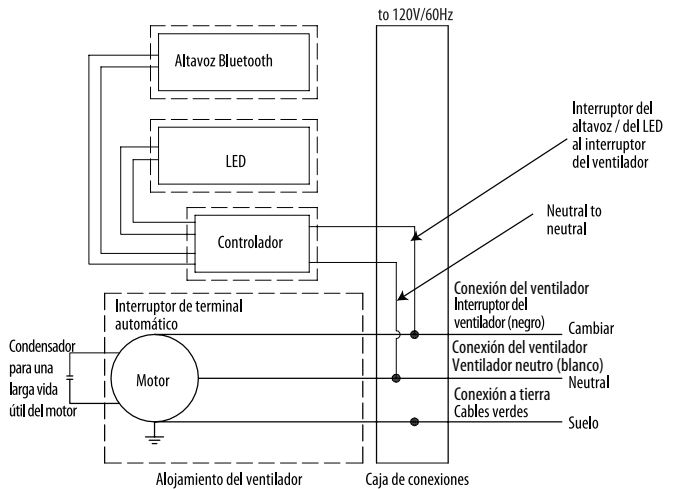
CABLEADO PARA 1 OPERACIÓN DE INTERRUPTOR
