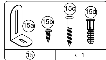
⑮ x 1 #A84050 safety bracket kit juego del soporte de seguridad ensemble de courroie de sécurité
