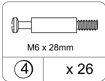
CAM BOLT Tornillo de rosca TDK0001
