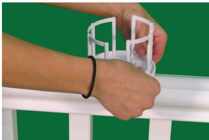
Snap wind guards into base Encaje los protectores contra el viento en la base
