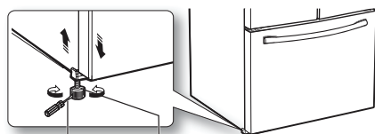
Tournevis à lame plate (-) Molette plate (-)
