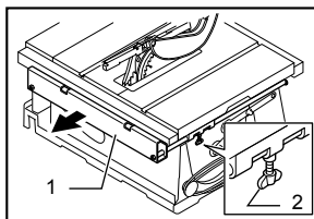
1. Submesa (posterior) 2. Tornillo
