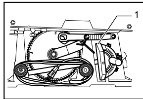
1. Calibrador de ingletes
