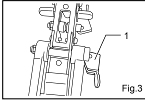
1. La palanca sujetadora en posición asegurada
