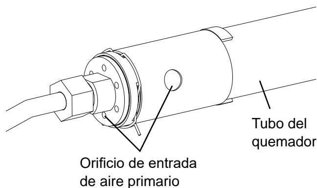
Fig. 24 - Ranura de entrada de aire primario en el tubo del quemador
