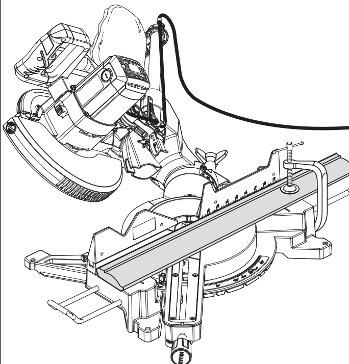
COUPE D'ONGLET COMPOSÉ 45° X 45°
