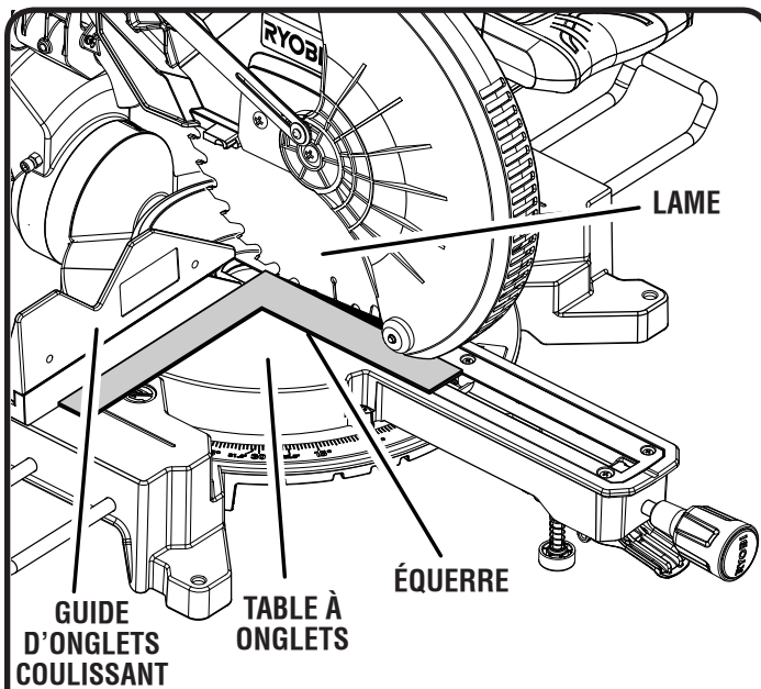
VUE DE LA LAME PAS D'ÉQUERRE AVEC LE GUIDE, DES RÉGLAGES SONT NÉCESSAIRES Fig. 21
