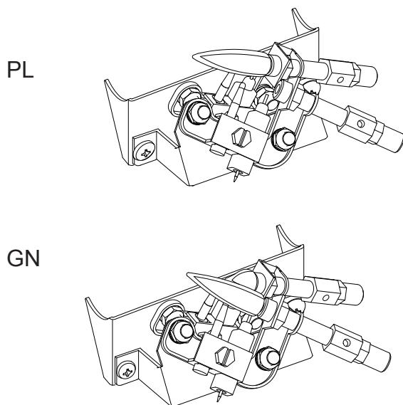
Fig. 26 - Patrón correcto de llama piloto
