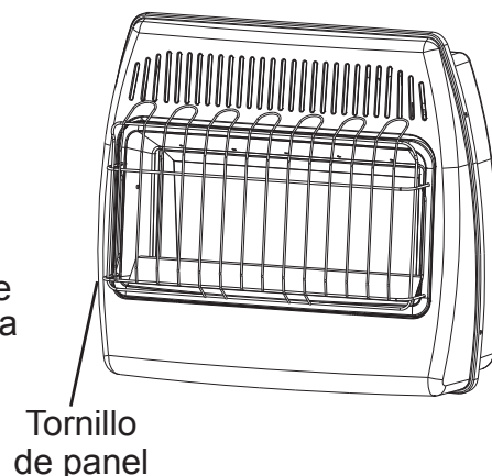
Fig. 30 - Retiro del panel frontal
