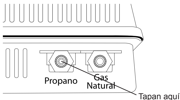
Fig. 5a - El ubicación de la clavija reguladora
