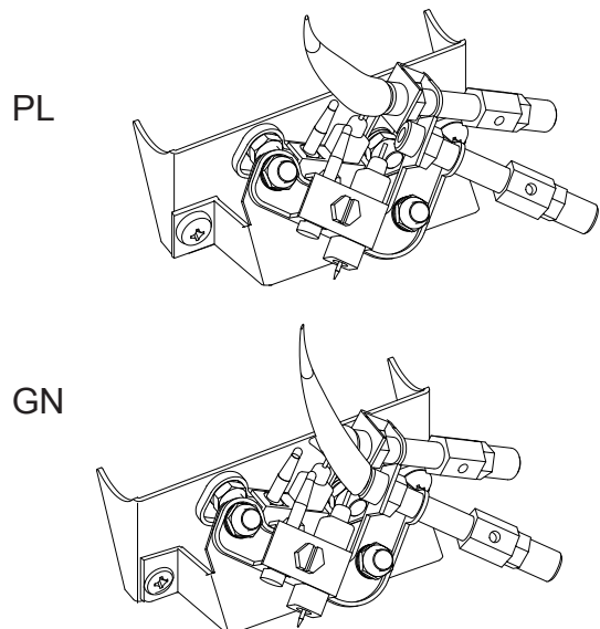
Fig. 27 - Patrón incorrecto de llama piloto
