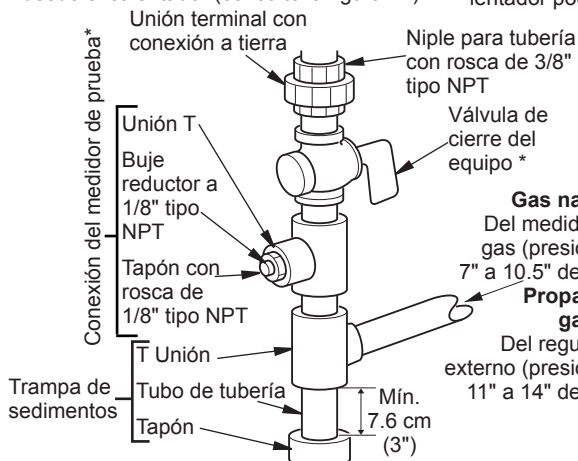
Figura 14 - Conexión de gas
