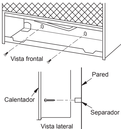
Figura 11 - Instalación de los tornillos de montaje inferiores
