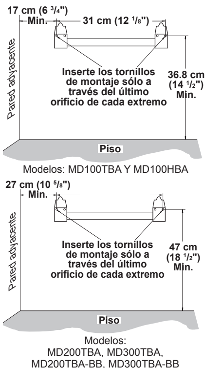
Figura 7 - Distancias mínimas del soporte de montaje
