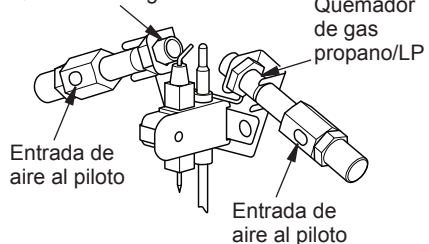
Figura 26 - Orificio de entrada de aire al piloto
