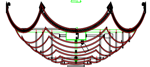
01-Lamp Body
